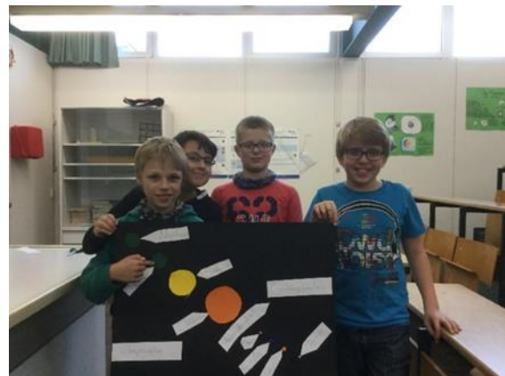
Unsere Übersicht zum Aufbau des Sonnensystems
